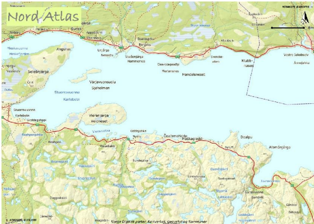
Kárta 2. Kárttas oaidná enaš oasi mu dutkanguovllus, njárgaid, vuonaid, sulluid ja giláziid. Buoret gova lea vejolaš oažžut jus geavaha neahttabáikki nordatlas.no ja zooma Várjavuona siskkimuš oasi (Nordatlas).
